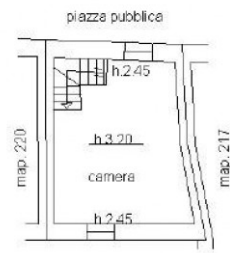
piano primo
