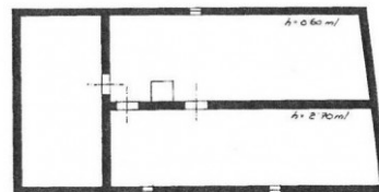
Pianta Piano Soffitta.
