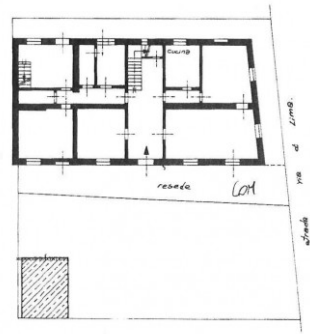
Pianta Piano Terra. A = 9,35 m 2
